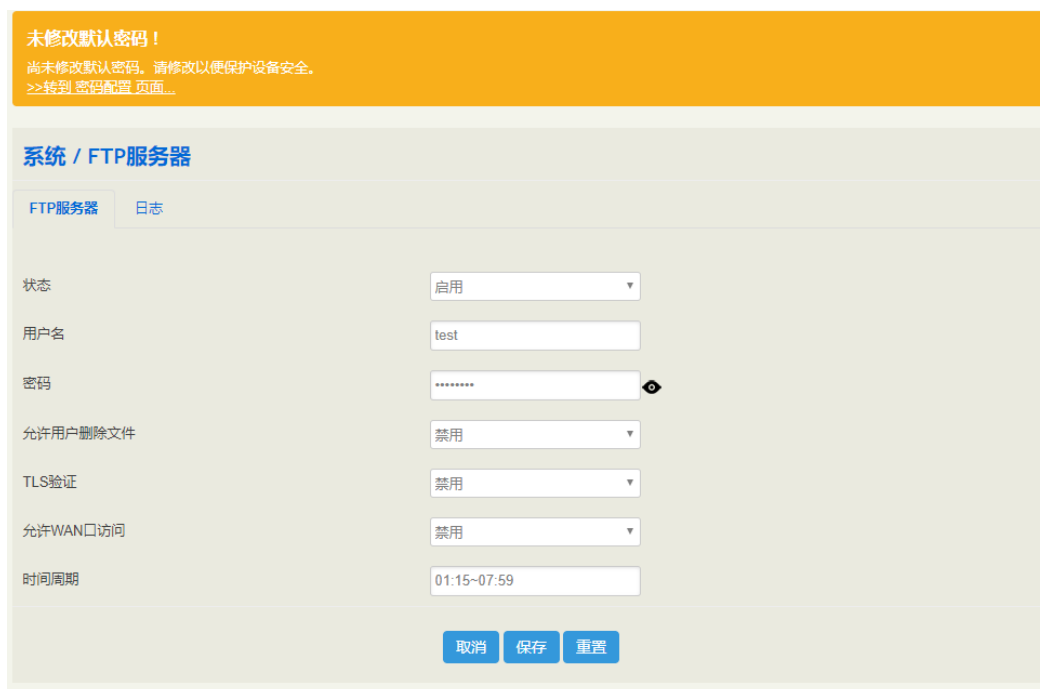
图 5-34 FTP 服务器
