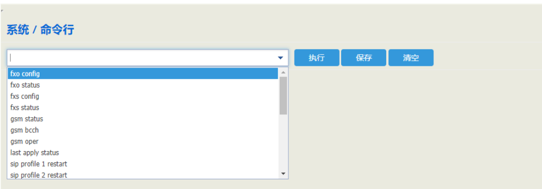
图 5-24 命令行
